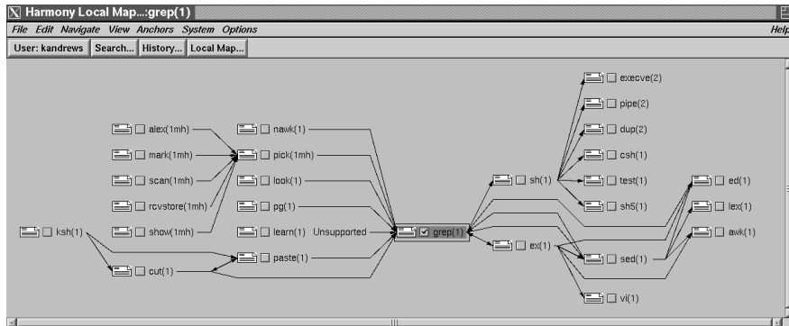
Fig. 6.: Harmony local map
